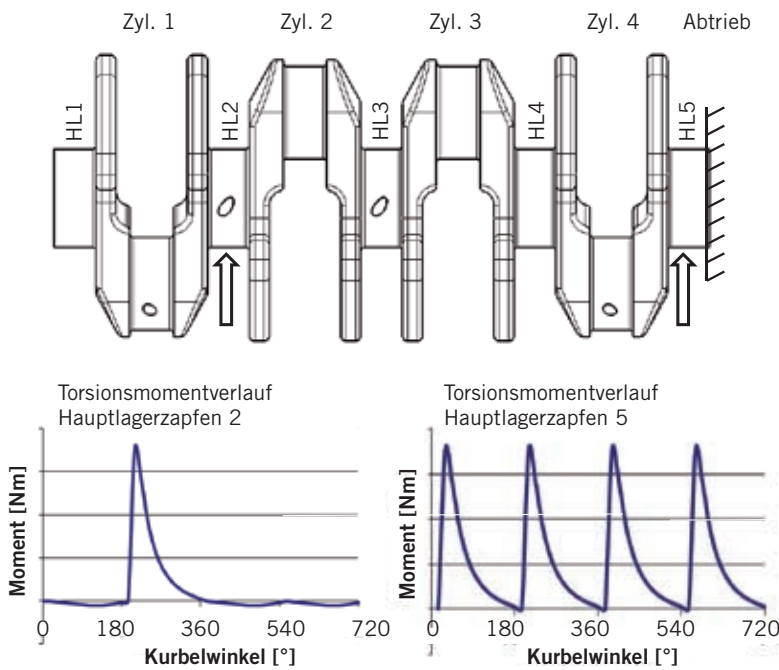
2 Schematische Torsionsmomentverläufe in unterschiedlichen Hauptlagerzapfen
